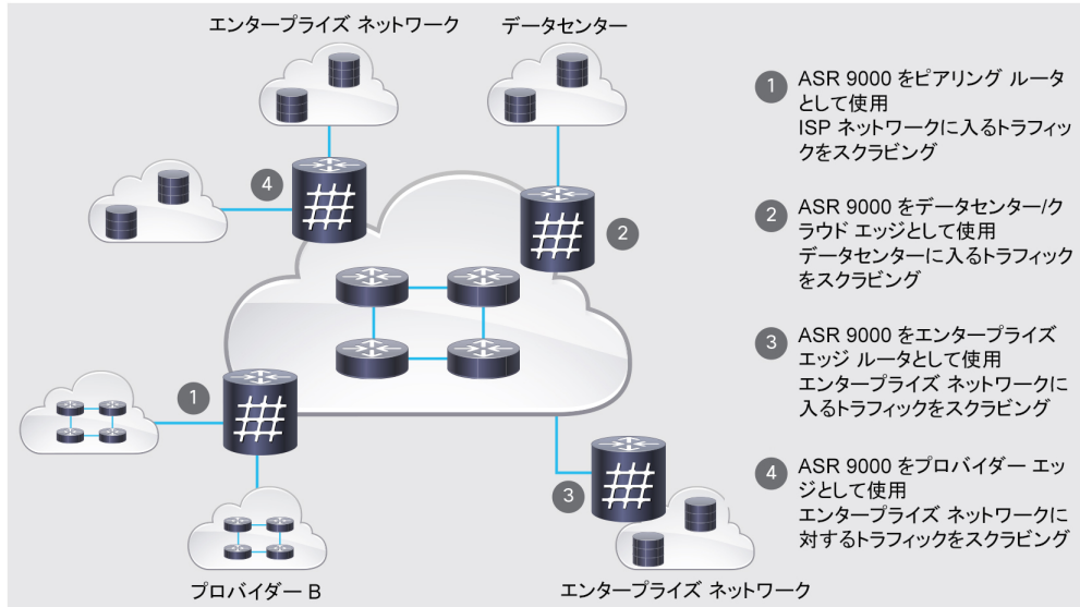
図 1. ASR 9000 vDDoS 攻撃対策ソリューションの配置
