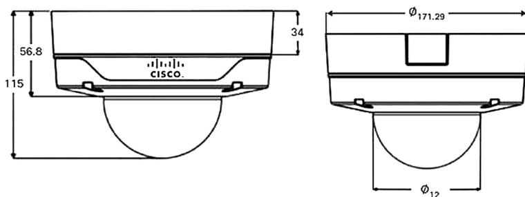
図 1. Cisco Video Surveillance 3620 および 3630 IP カメラの寸法
