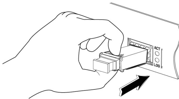
Figura 7: Installazione di un modulo ricetrasmittitore
