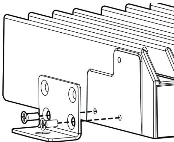
Figura 6: Fissaggio del kit per montaggio a parete
