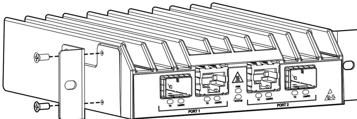
Figura 7: Fissaggio delle staffe di montaggio a L
