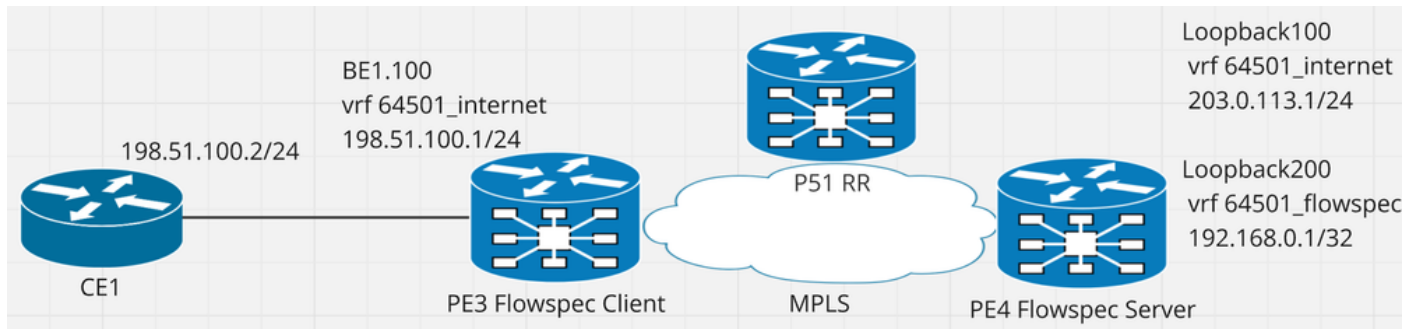
Figura 1: diagramma reticolare con gli indirizzi IP pertinenti.
