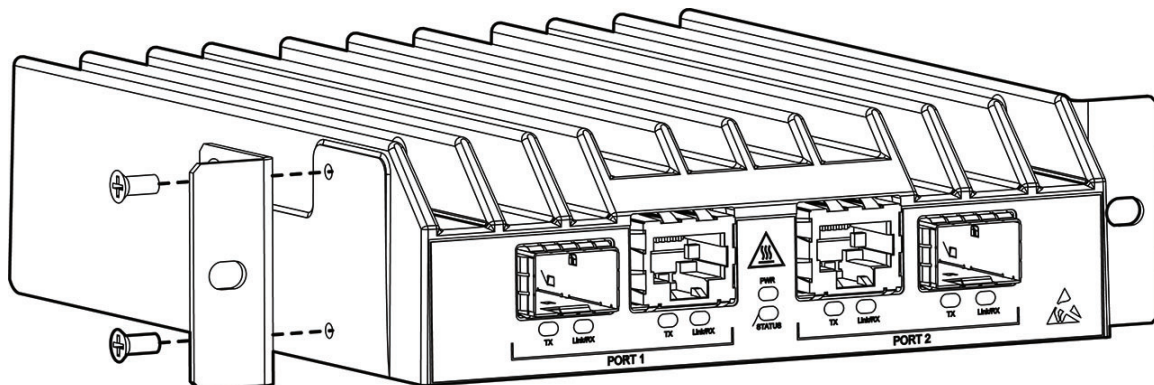
Illustration 2 : Fixer les supports de montage en L
