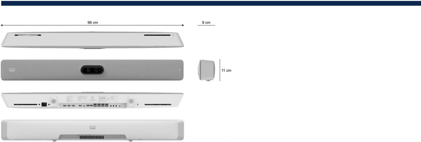
Figure 4. L'unité de barre vidéo Cisco Room Bar Pro vue de haut, devant, côté, bas et arrière
