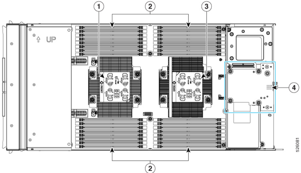
Illustration 3 : Nœud de traitement informatique Cisco UCS X410c M8, secondaire, couche supérieure
