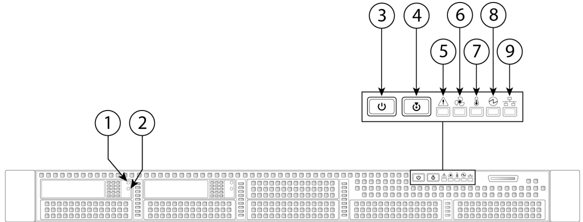
Illustration 3 : Voyants DEL du panneau avant et leurs états
