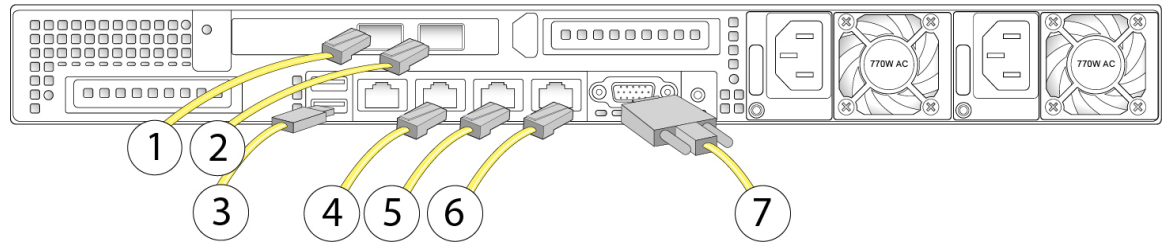
Illustration 7 : Connexions des câbles
