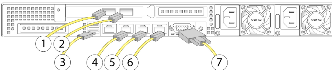
Illustration 5 : Connexions des câbles
