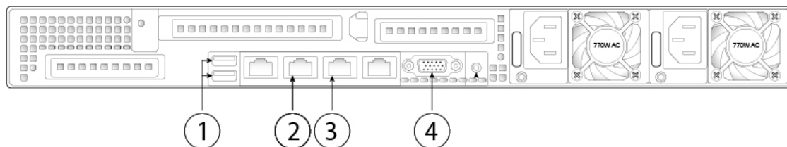
Illustration 1 : Panneau arrière de FMC 1000
