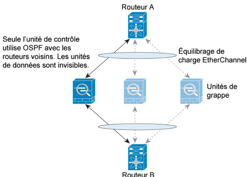
Illustration 9 : Routage dynamique
