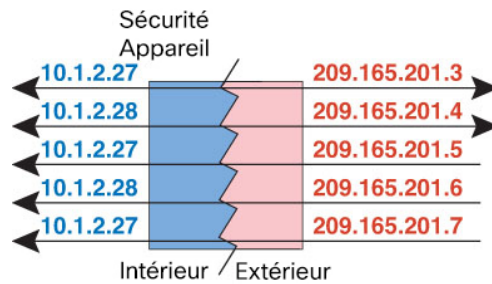
Illustration 37 : NAT statique quelques-uns vers plusieurs
