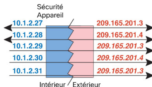
Illustration 38 : NAT statique plusieurs à quelques-uns
