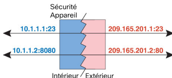
Illustration 34 : NAT statique typique avec scénario de traduction de port
