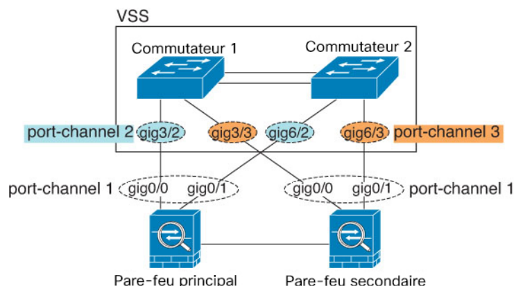
Illustration 8 : Basculement actif/en veille et VSS/vPC
