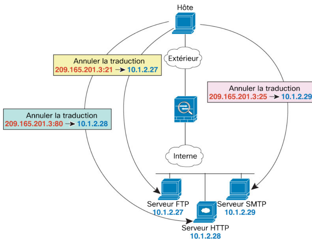
Illustration 41 : NAT statique avec traduction de port
