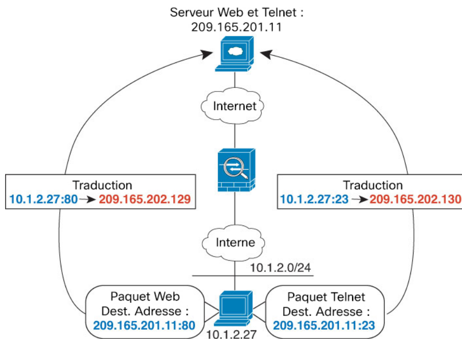
Illustration 43 : NAT manuelle avec différents ports de destination
