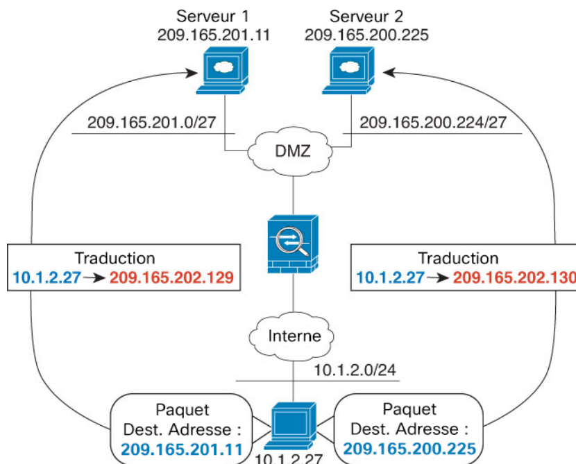
Illustration 42 : NAT manuelle avec différentes adresses de destination
