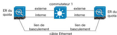
Illustration 5 : Connexion avec un câble
