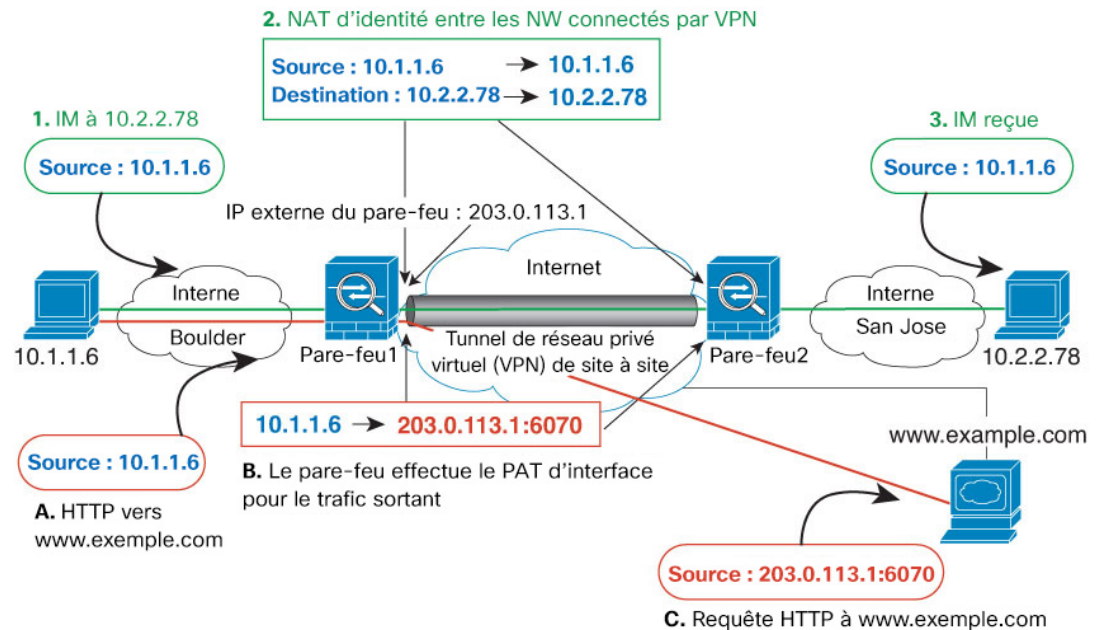
Illustration 44 : PAT d'interface et NAT d'identité pour le VPN de site à site
