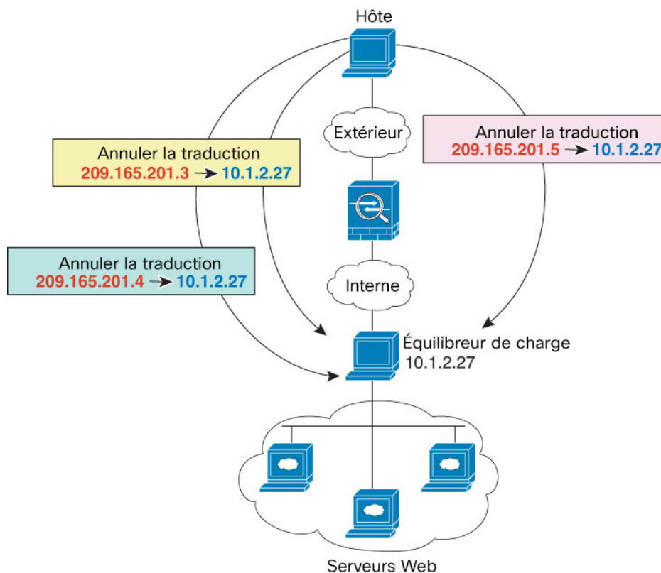
Illustration 36 : Exemple de NAT statique un vers plusieurs
