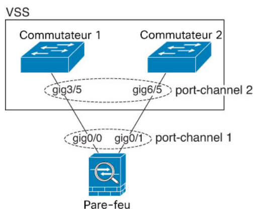
Illustration 7 : Connexion à un VSS/vPC
