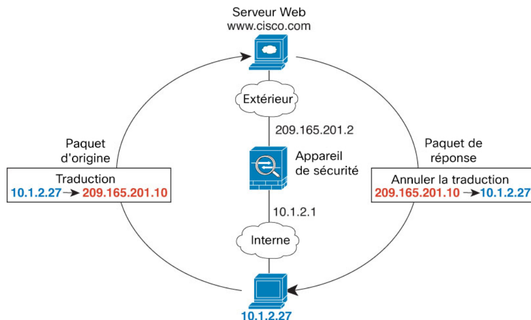
Illustration 28 : Exemple de NAT : mode routé
