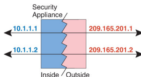
Illustration 6 : NAT statique
