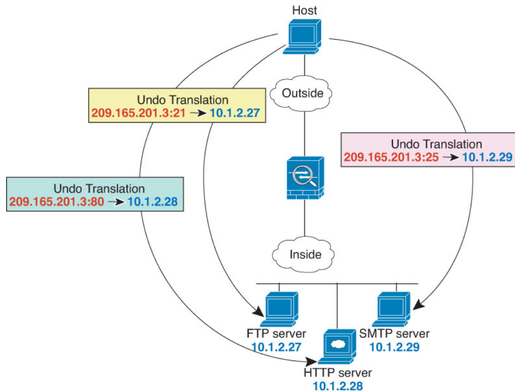
Illustration 14 : NAT statique avec traduction de port
