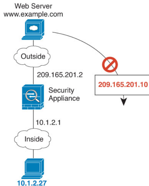
Illustration 4 : L'hôte distant tente d'établir une connexion à une adresse mappée
