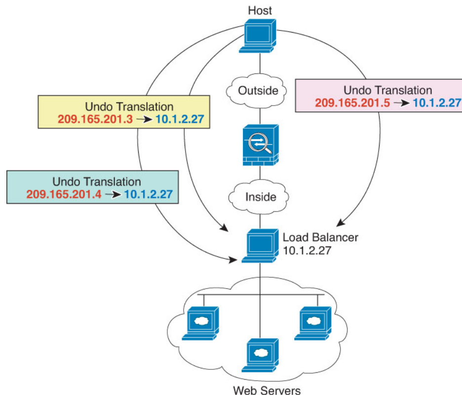
Illustration 9 : Exemple de NAT statique un vers plusieurs
