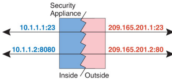
Illustration 39 : NAT statique typique avec scénario de traduction de port
