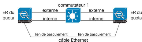
Illustration 10 : Connexion avec un câble
