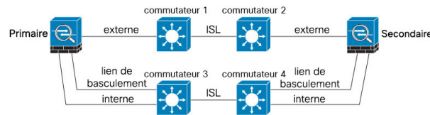
Illustration 11 : Connexion avec un commutateur sécurisé
