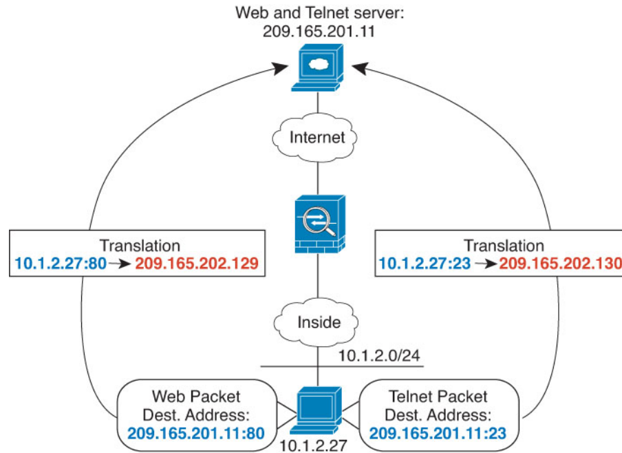
Illustration 48 : NAT manuelle avec différents ports de destination
