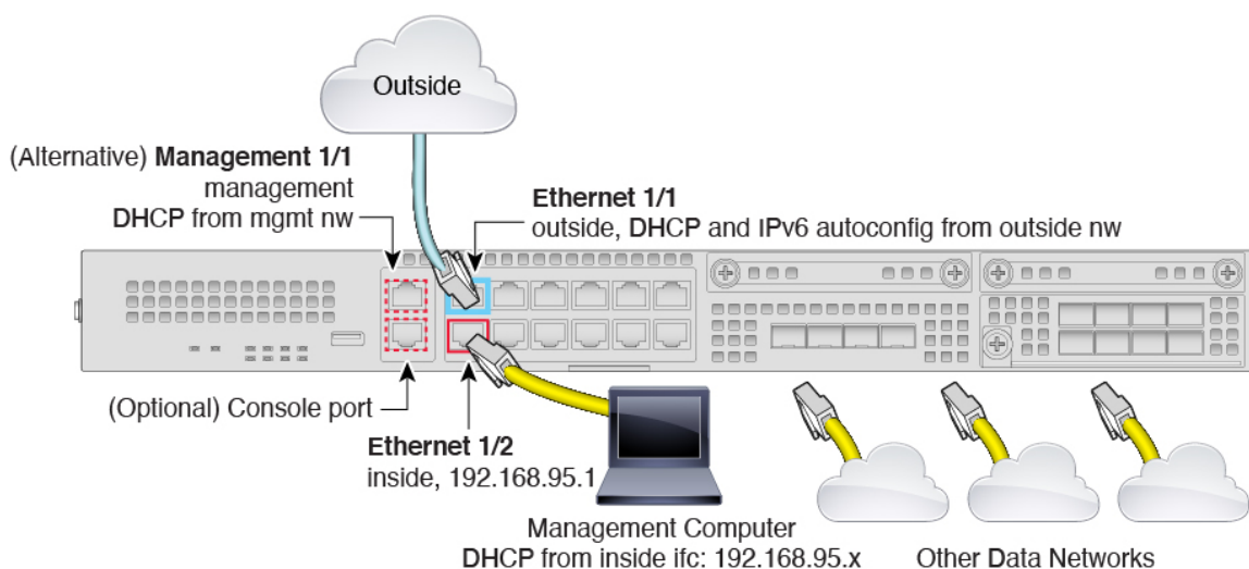
Illustration 3 : Câblage du Firepower 2100
