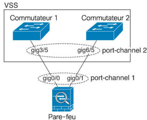
Illustration 12 : Connexion à un VSS/vPC
