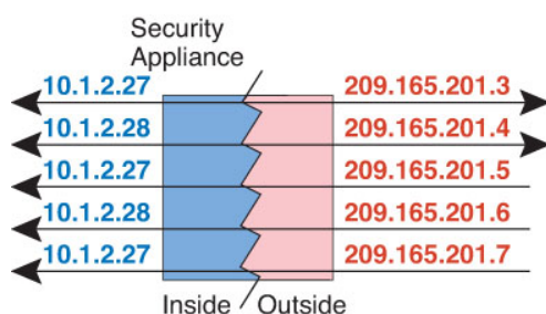
Illustration 42 : NAT statique quelques-uns vers plusieurs
