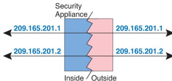
Illustration 44 : NAT d'identité
