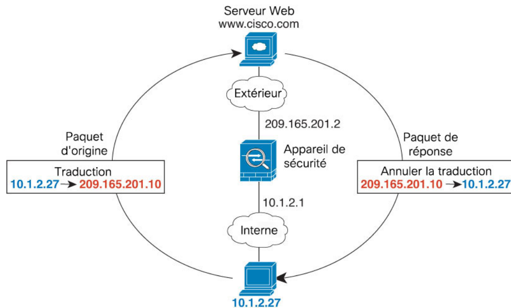
Illustration 33 : Exemple de NAT : mode routé
