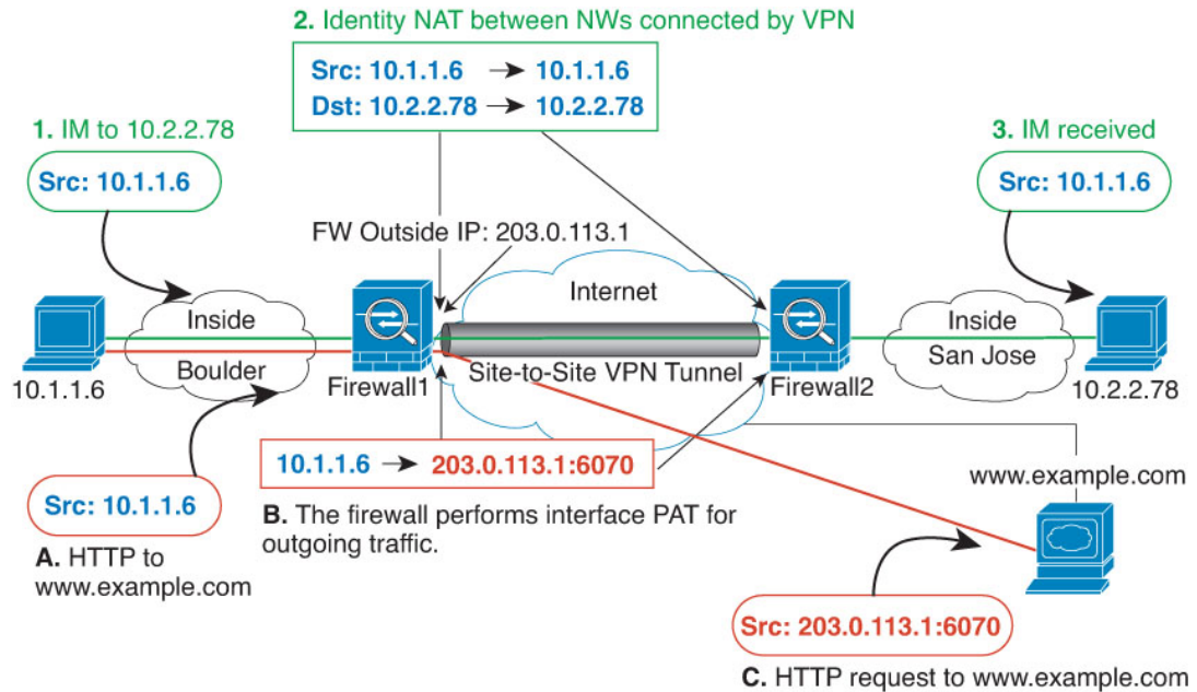
Illustration 49 : PAT d'interface et NAT d'identité pour le VPN de site à site
