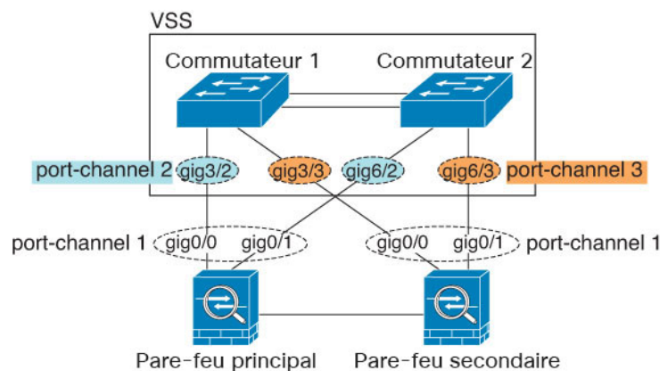
Illustration 13 : Basculement actif/en veille et VSS/vPC
