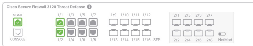
Illustration 20 : Activer le module de réseau
