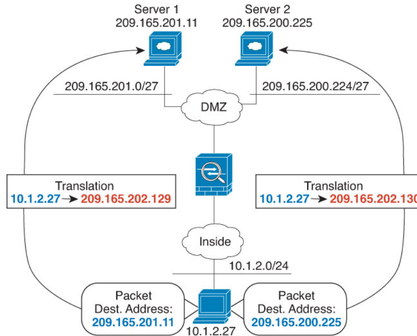
Illustration 47 : NAT manuelle avec différentes adresses de destination
