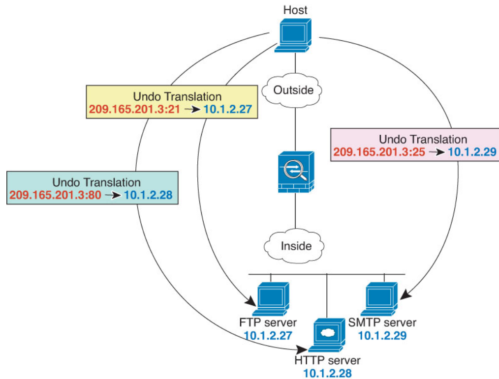
Illustration 46 : NAT statique avec traduction de port
