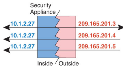
Illustration 40 : NAT statique un vers plusieurs
