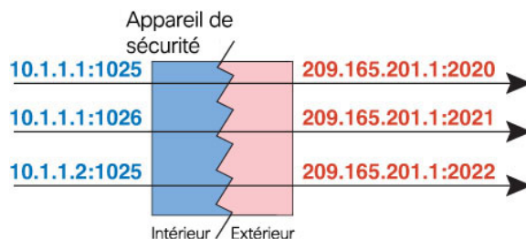
Illustration 37 : PAT dynamique
