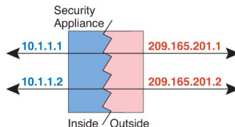
Illustration 38 : NAT statique
