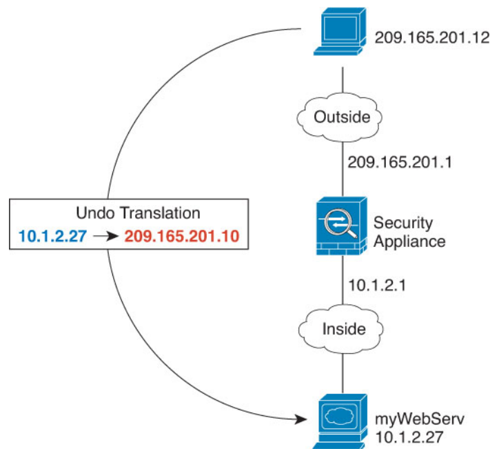
Illustration 45 : NAT statique pour un serveur Web interne
