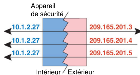
Illustration 8 : NAT statique un vers plusieurs
