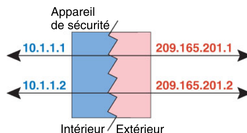
Illustration 6 : NAT statique
