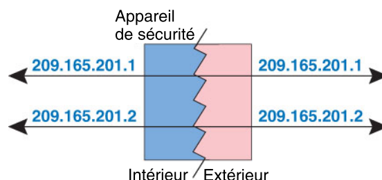
Illustration 12 : NAT d'identité
