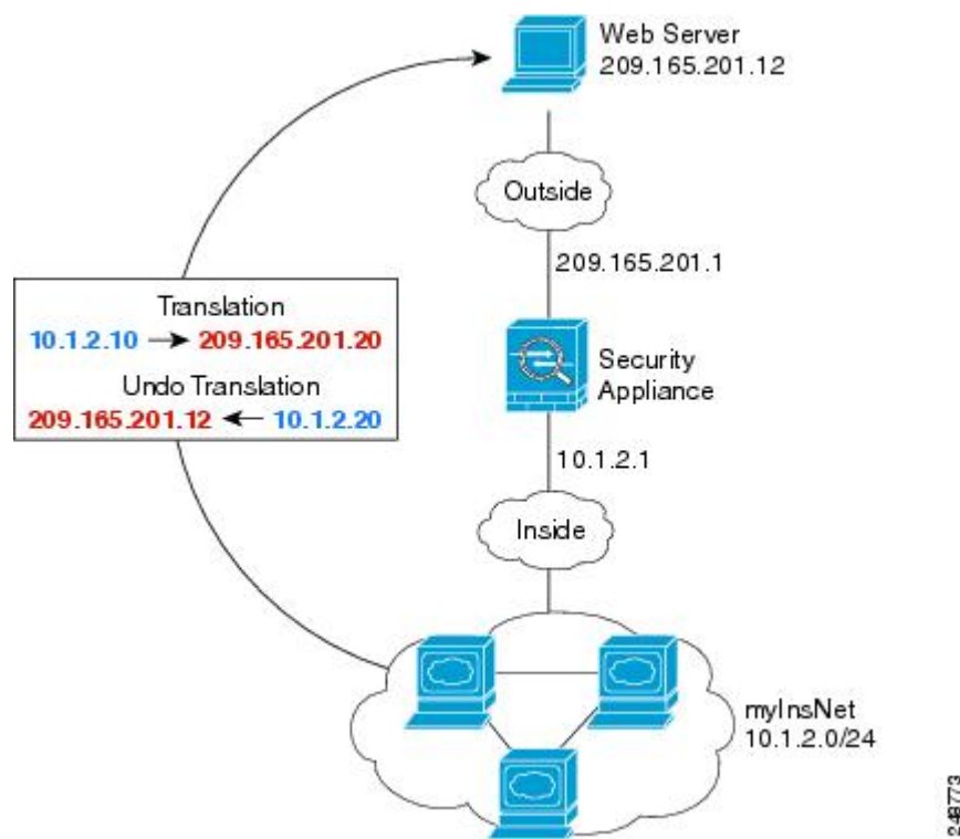
Illustration 2 : NAT dynamique pour l'interne, NAT statique pour le serveur Web externe
