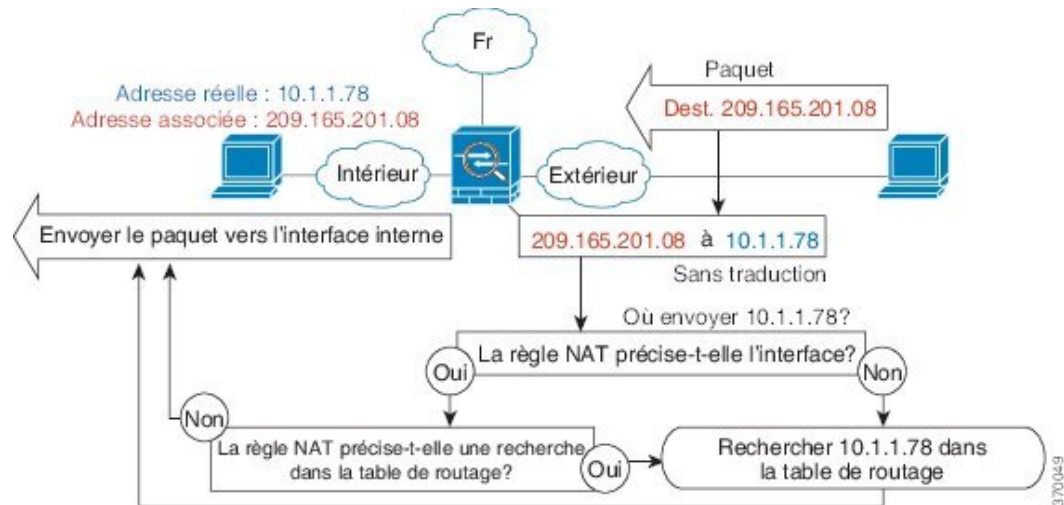
Illustration 11 : Sélection de l'interface de sortie en mode routé avec NAT
