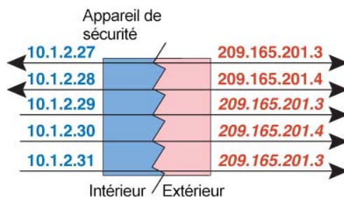
Illustration 10 : NAT statique plusieurs à quelques-uns
