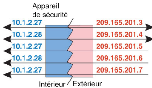
Illustration 9 : NAT statique quelques-uns vers plusieurs
