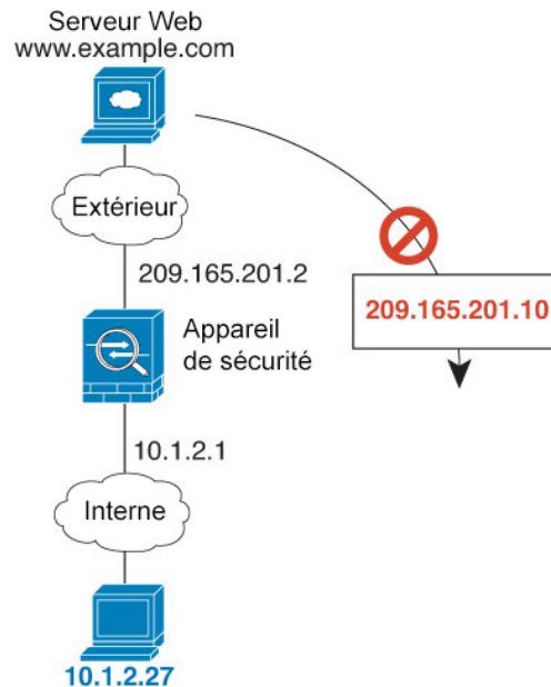
Illustration 3 : L'hôte distant tente d'établir une connexion à une adresse mappée
