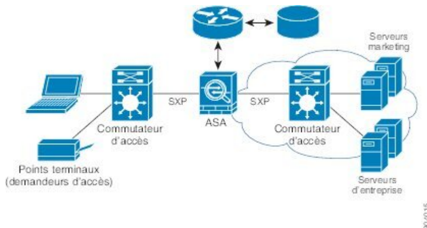
Illustration 1 : Déploiement de l'application des politiques basées sur le nom de groupe de sécurité
