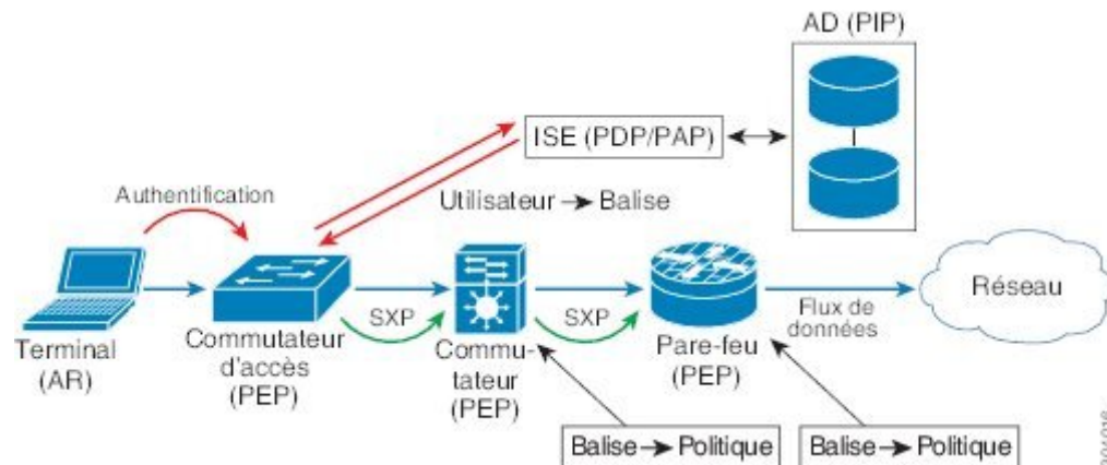
Illustration 2 : Application de la politique de sécurité
