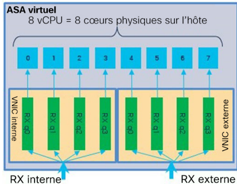
Illustration 4 : Files d'attente RX RSS à 8 cœurs ASA virtuel
