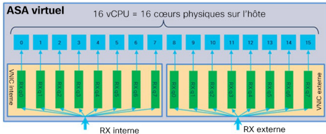
Illustration 5 : Files d'attente RX RSS à 16 cœurs ASA virtuel
