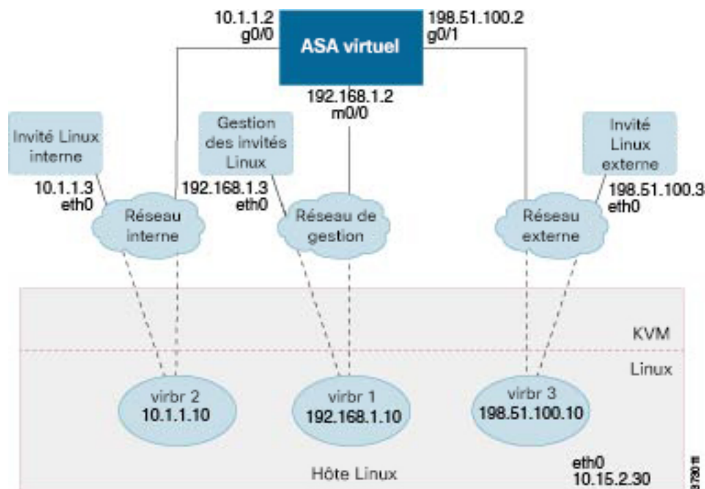
Illustration 1 : Exemple de déploiement d'ASA virtuel à l'aide de KVM
