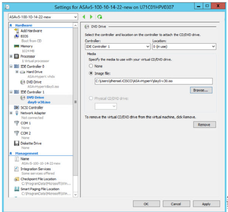
Illustration 2 : Gestionnaire Hyper-V
