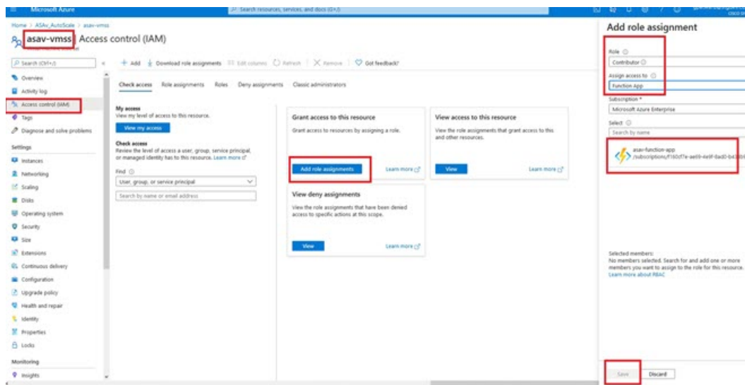
Illustration 12 : Affectation du rôle AIM
