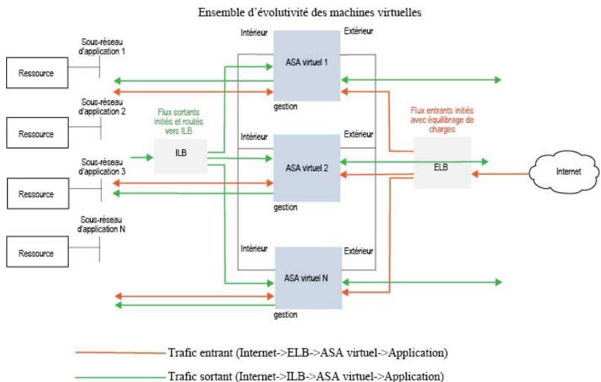
Illustration 1 : Scénario d'évolutivité automatique ASA virtuel
