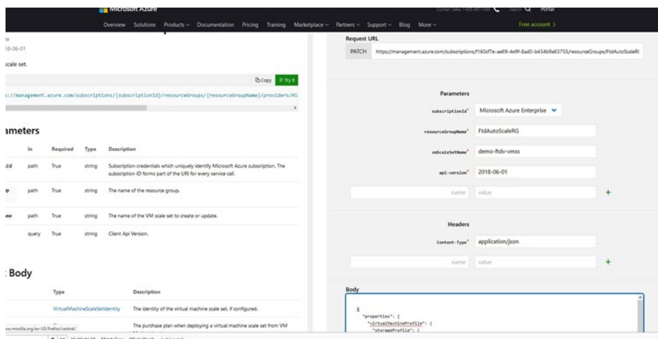
Illustration 17 : Mettre à niveau l'ASA virtuel
