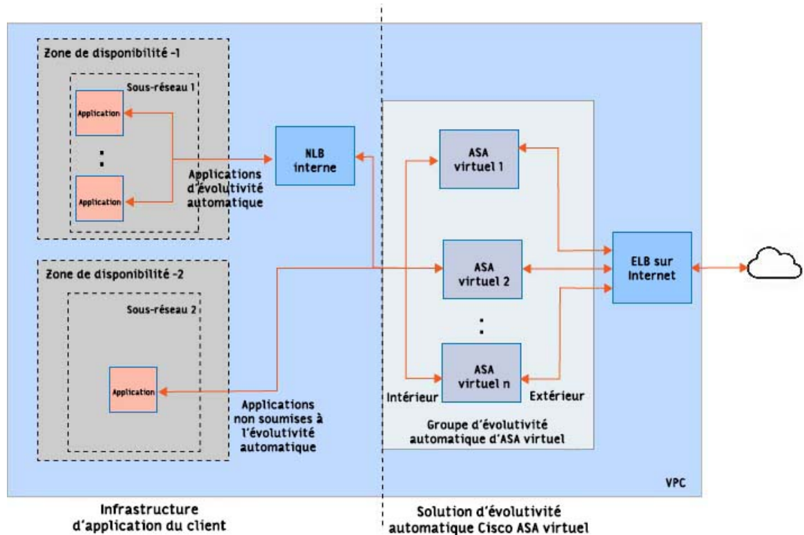
Illustration 1 : Diagramme des scénarios d'évolutivité automatique d'ASA virtuel
