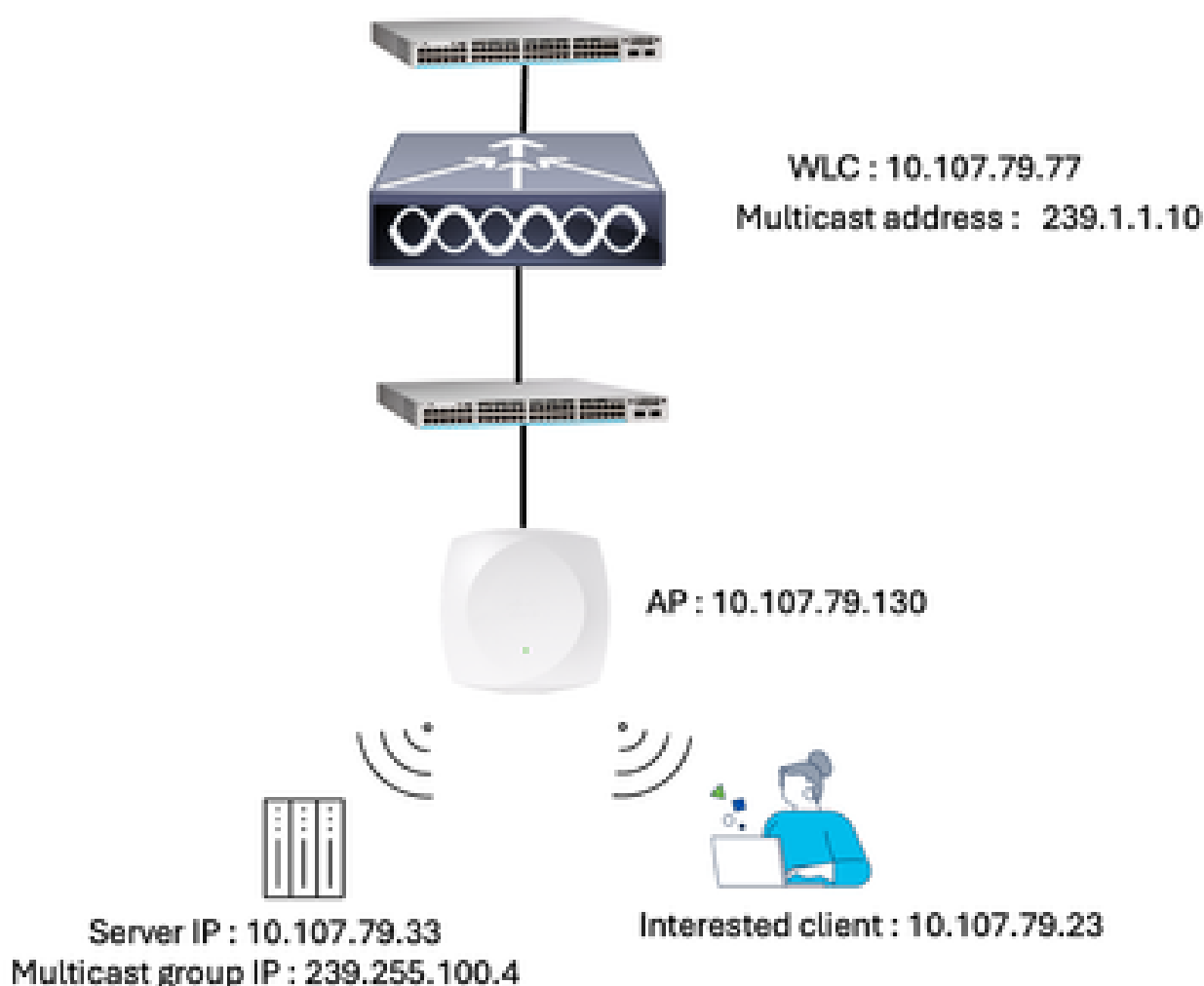
Diagramme du réseau
