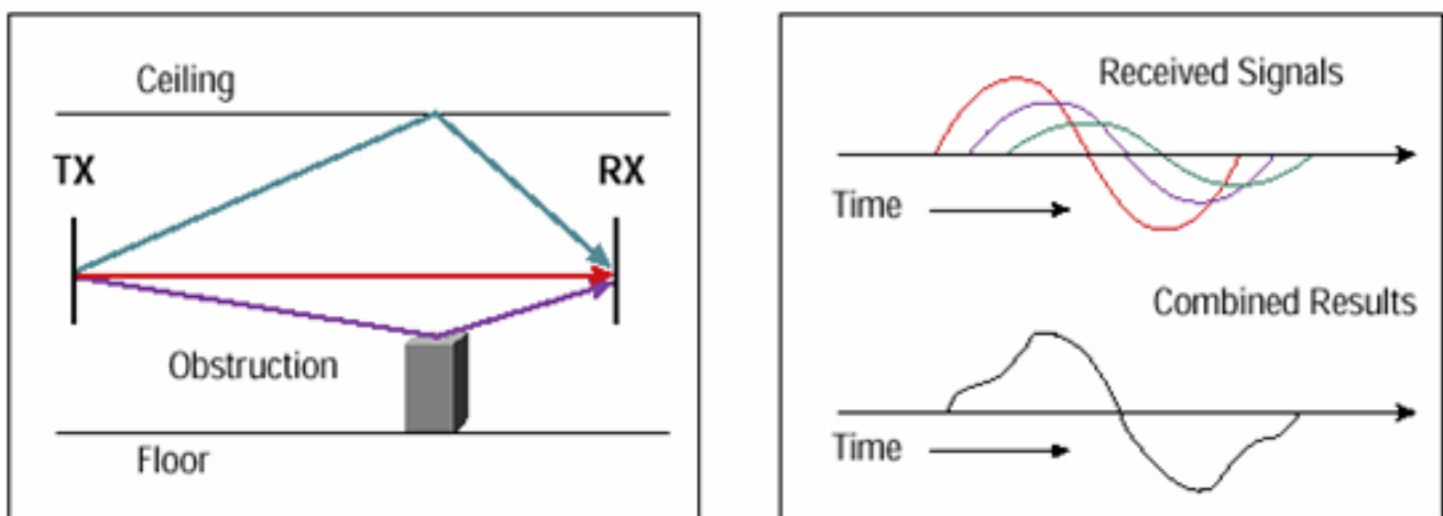
Figure 7 : Effets des trajets multiples sur l'environnement intérieur
