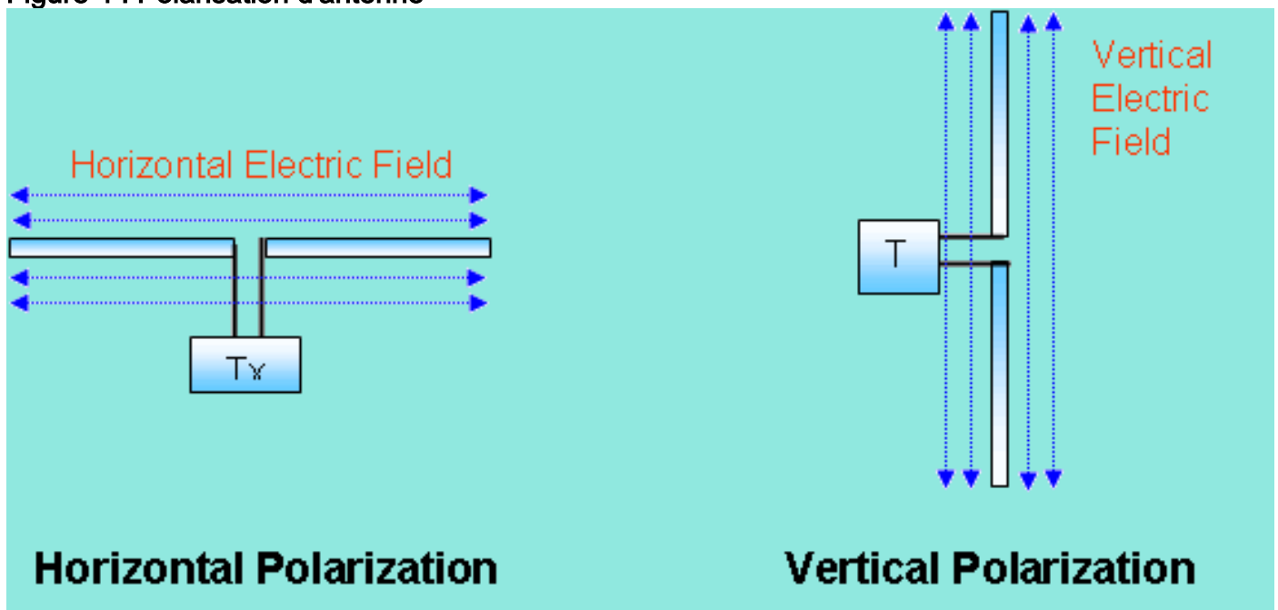
Figure 4 : Polarisation d'antenne
