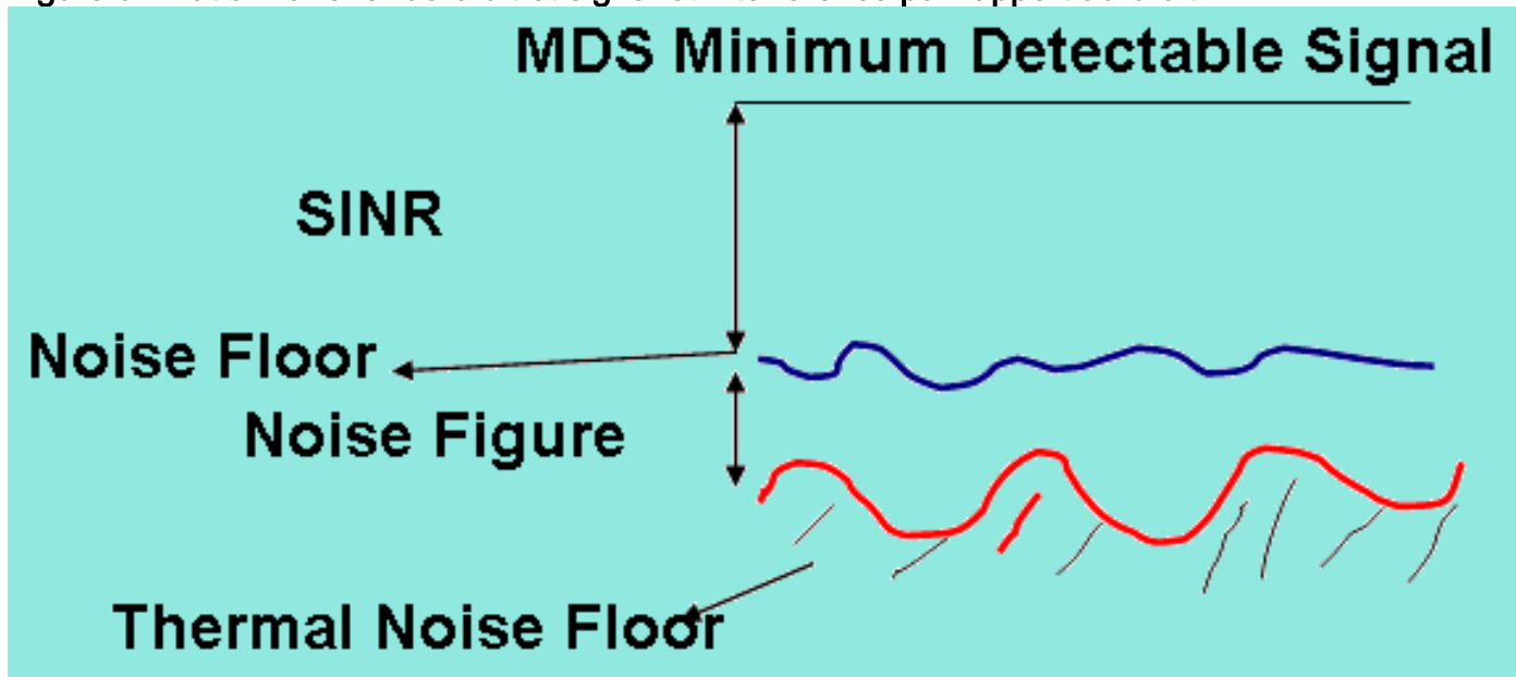
Figure 9 : Ratio Plancher de bruit et signal et interférence par rapport au bruit
