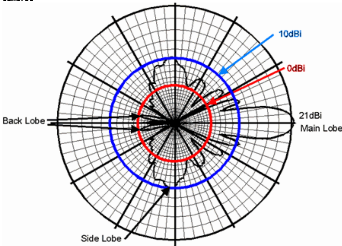
Figure 6 : Diagramme de rayonnement habituel d'une antenne directionnelle avec des lobes calibrés
