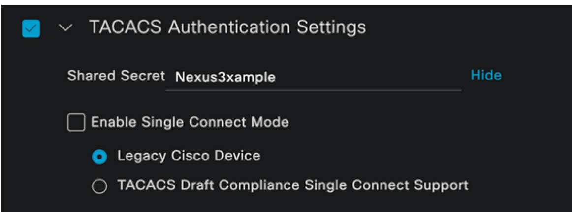
Section de configuration TACACS
