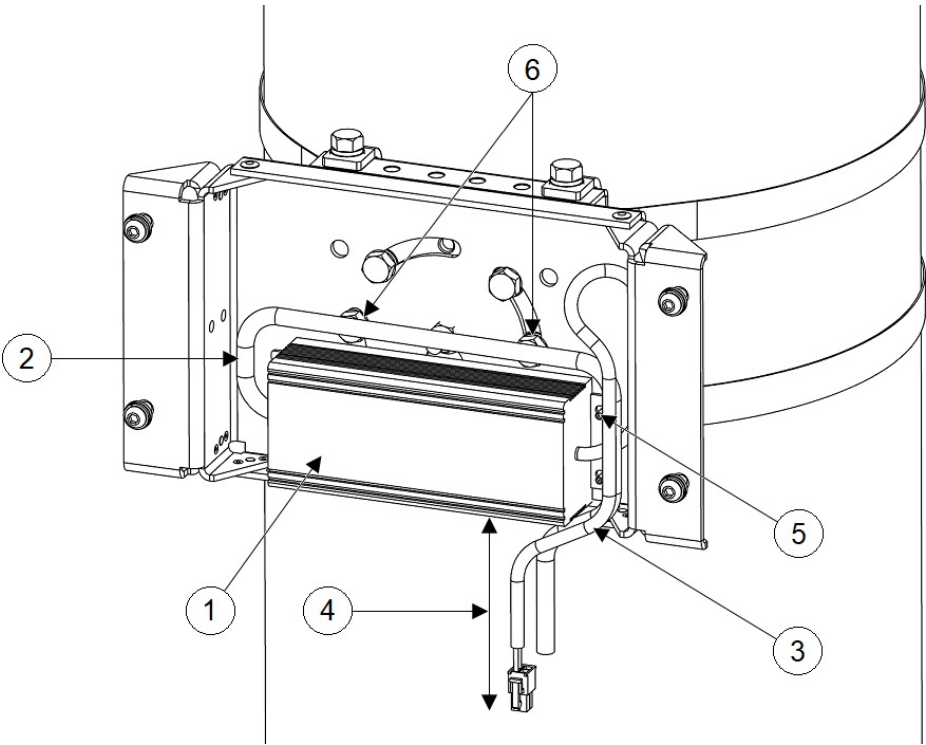
Figura 13: Adaptador de alimentación instalado con el soporte de montaje AIR-ACCPMK3700-2=
