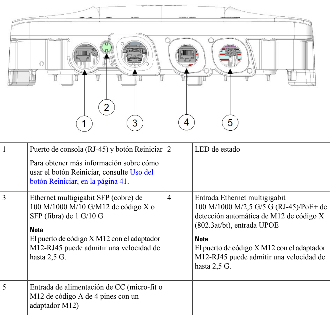
Figura 1: Conectores y puertos del panel frontal del IW91671
