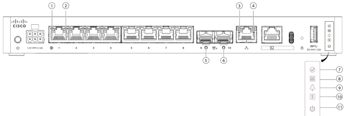
Figura 10: Indicadores LED del panel posterior de CSF-1220CX
