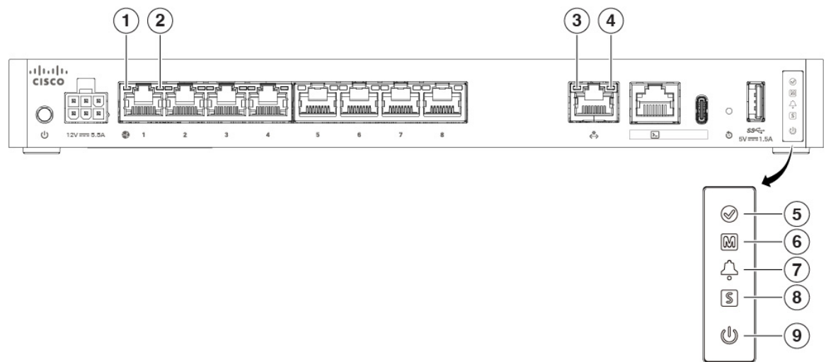
Figura 8: Indicadores LED del panel posterior de CSF-1210C
