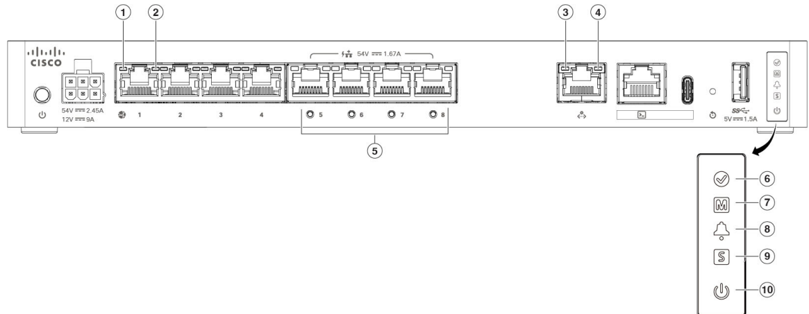
Figura 9: Indicadores LED del panel posterior de CSF-1210CP
