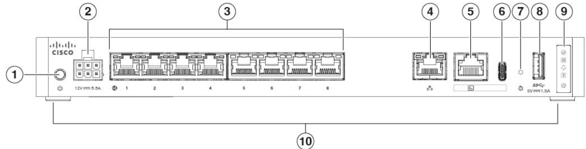
Figura 5: Panel posterior de CSF-1210CE
