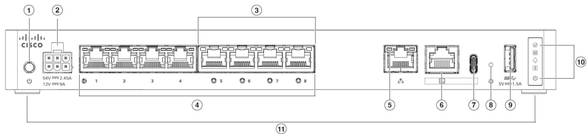
Figura 6: Panel posterior de CSF-1210CP
