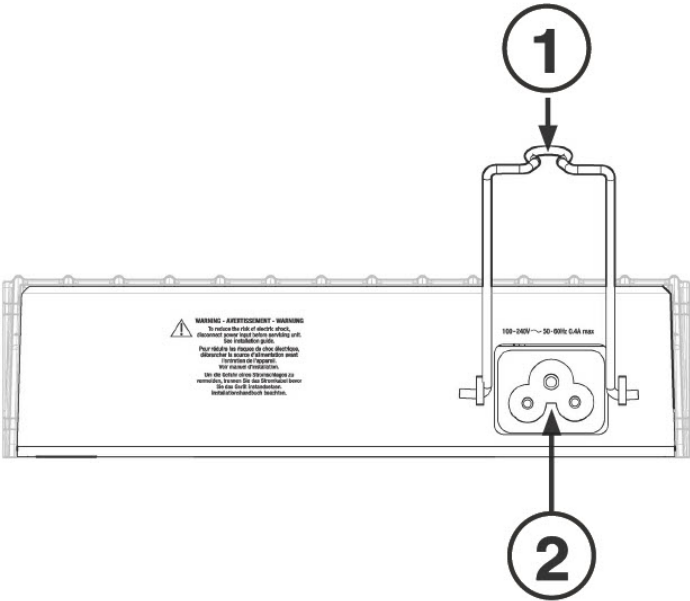
Figura 4: Panel posterior de Sensor Module 10G: modelo de alimentación de entrada de CA
