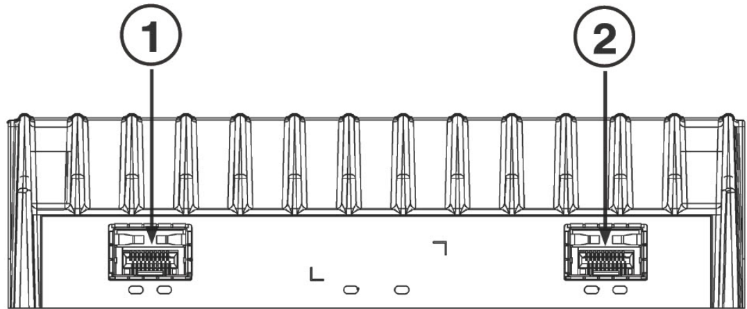
Figura 2: Panel frontal de Sensor Module 10G
