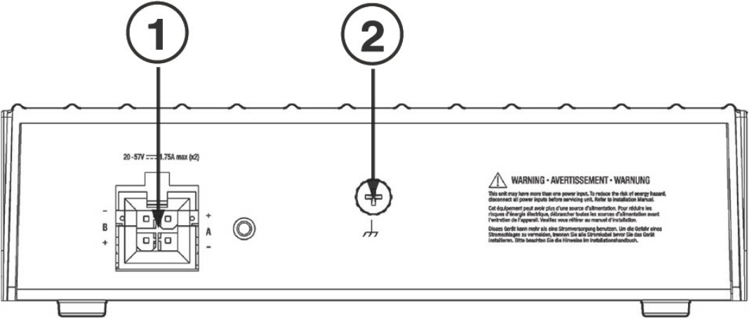
Figura 5: Panel posterior de Sensor Module 10G: modelo de alimentación de entrada de CC
