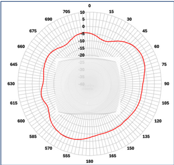
Figura 5. Patrones de antena de radio de IoT
