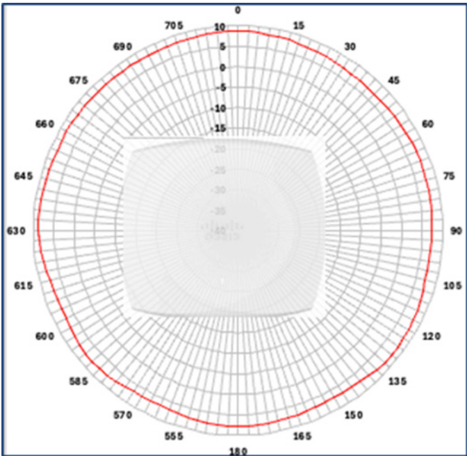
Figura 1. Patrones de antena
