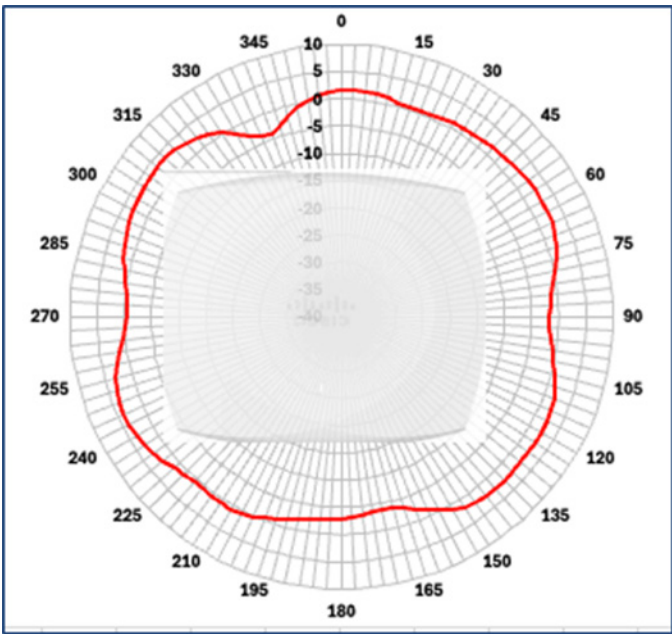
Figura 4. Patrones de antena de radio de escaneo impulsados por inteligencia artificial/ML
