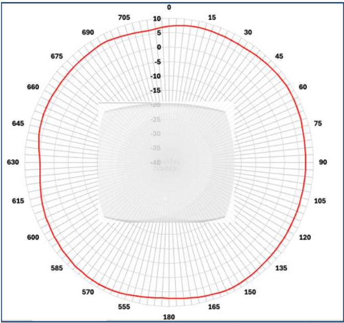
Figura 2. Patrones de antena de radio de 5 GHz de la ranura 2
