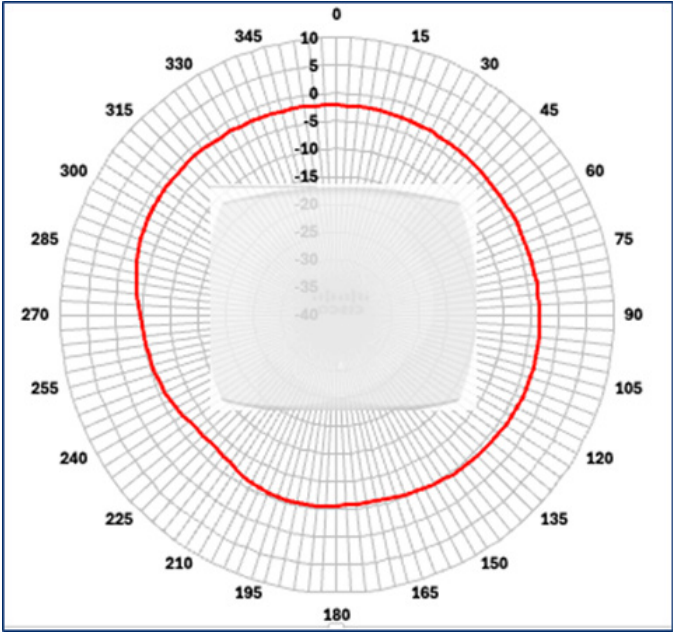
Figura 6. Patrones de antena GNSS
