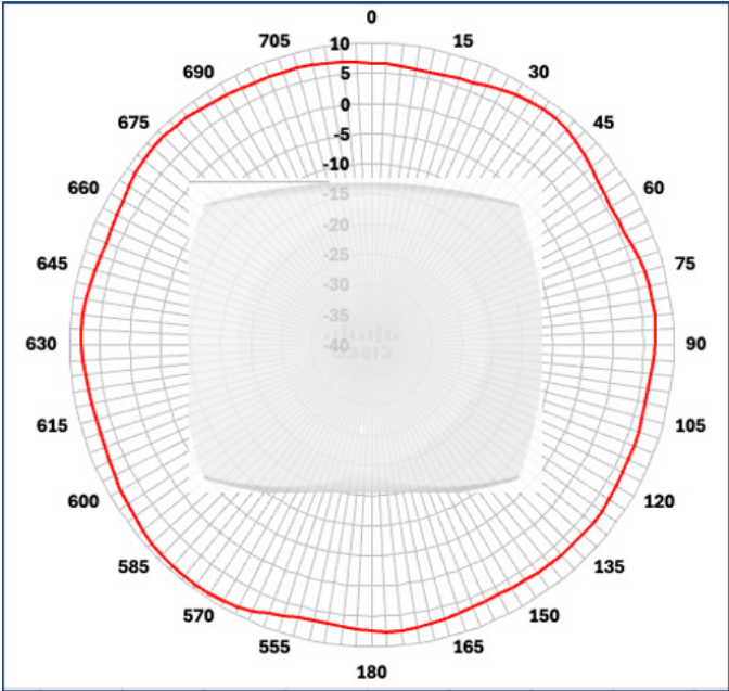
Figura 3. Patrones de antena de radio de 6 GHz
