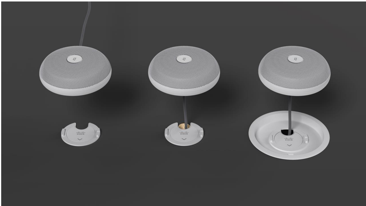
Figura 3. Opciones de montaje del Table Microphone Pro.
