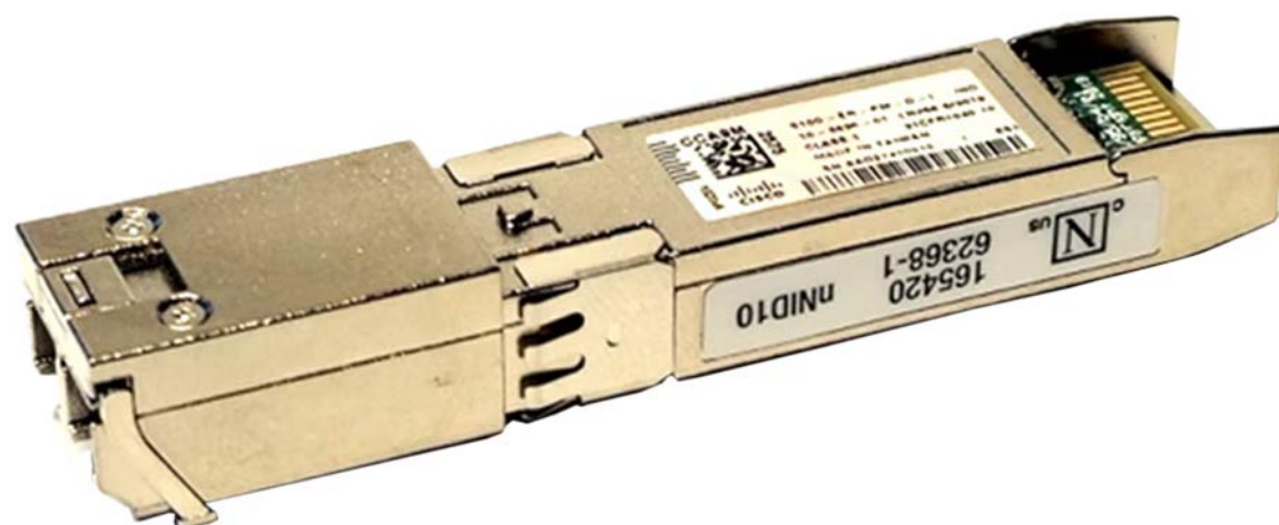
Figura 4: Transceptores bidireccionales de largo alcance (LR) 10 G (ascendente y descendente)
