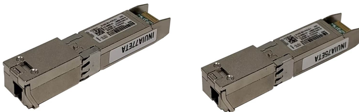
Figura 4: Transceptores bidireccionales de largo alcance (LR) 10 G (ascendente y descendente)
