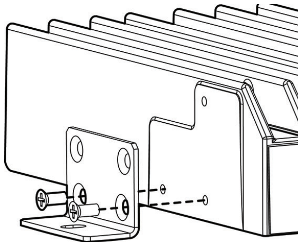
Figura 1: Fijación del kit de montaje en pared
