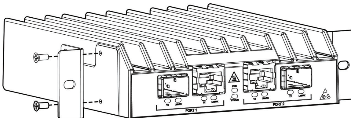
Figura 2: Fije los soportes de montaje en forma de L
