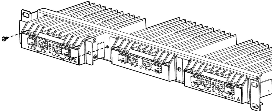
Figura 8: Deslizar el módulo
