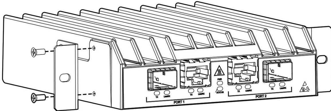
Figura 7: Fije los soportes de montaje en forma de L
