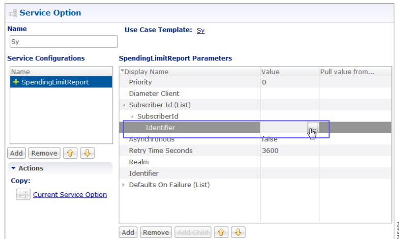
Figure 4: Identifier Parameter
