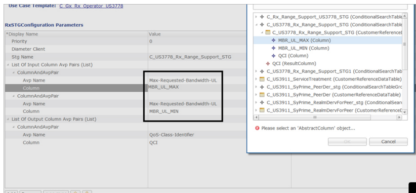
Figure 15: RxSTGconfiguration Column Parameter
