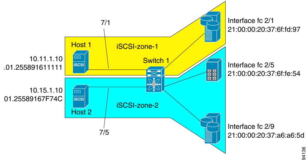
Figure 4-44 iSCSI Scenario 1
