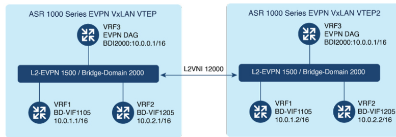
Figure 47: EVPN VxLAN on Layer 2 VTEP-2
