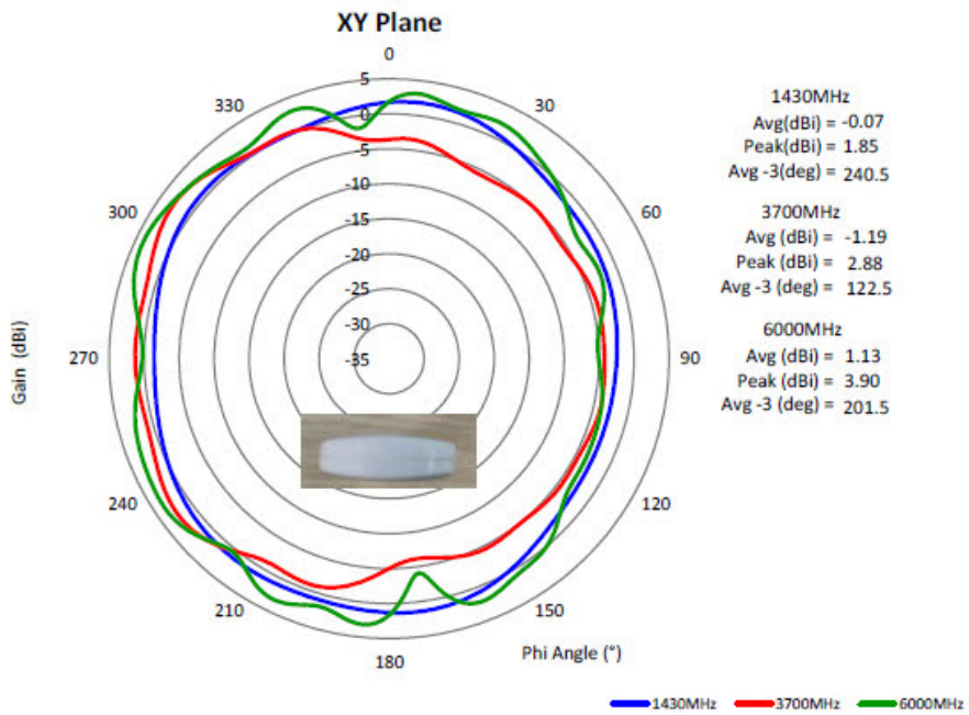
Gain Plots (bend) 1430-6000 MHz
