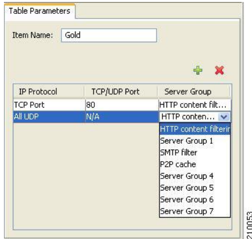
Figure 56: Tables Parameters Tab
