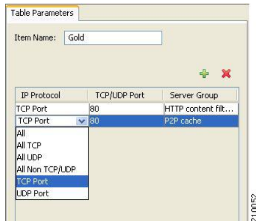
Figure 55: Table Parameters Tab
