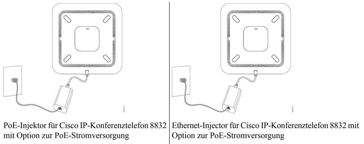
Abbildung 1: PoE-Stromversorgungsoptionen für Konferenztelefone
