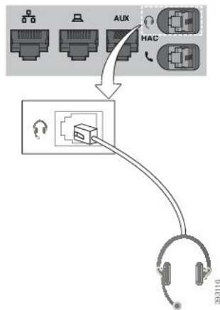
Abbildung 5: Standard-Headset-Verbindung
