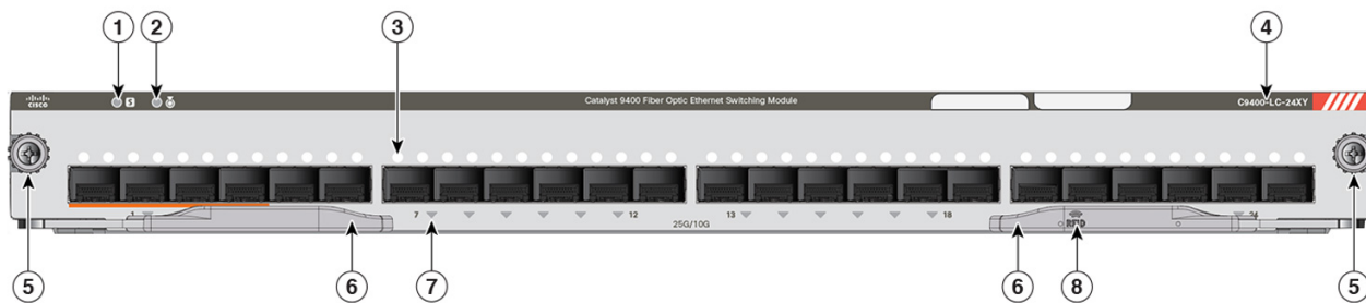
Abbildung 13: Vorderansicht der Linecard C9400-LC-24XY
