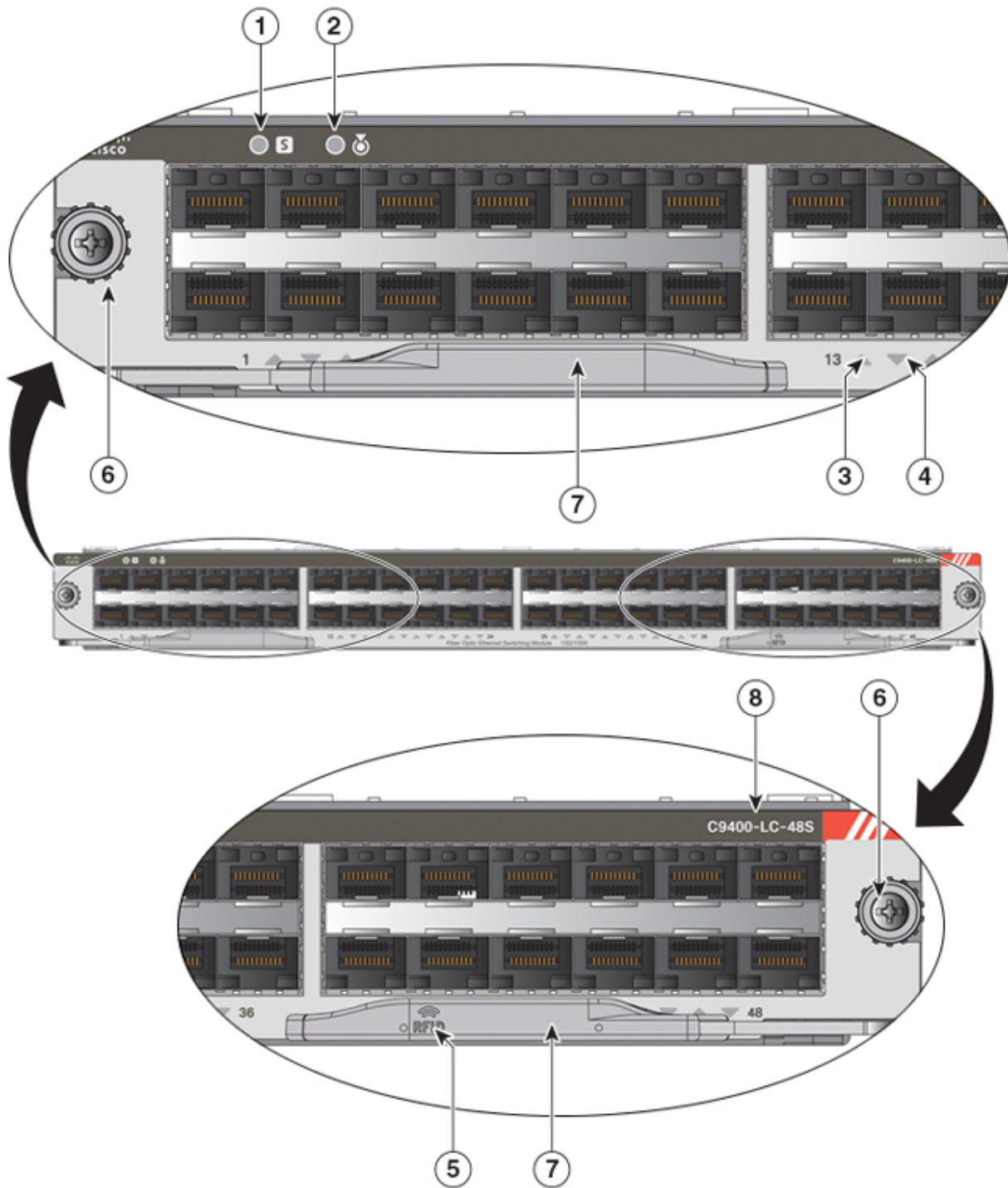
Abbildung 15: Vorderansicht der Linecard C9400-LC-48S
