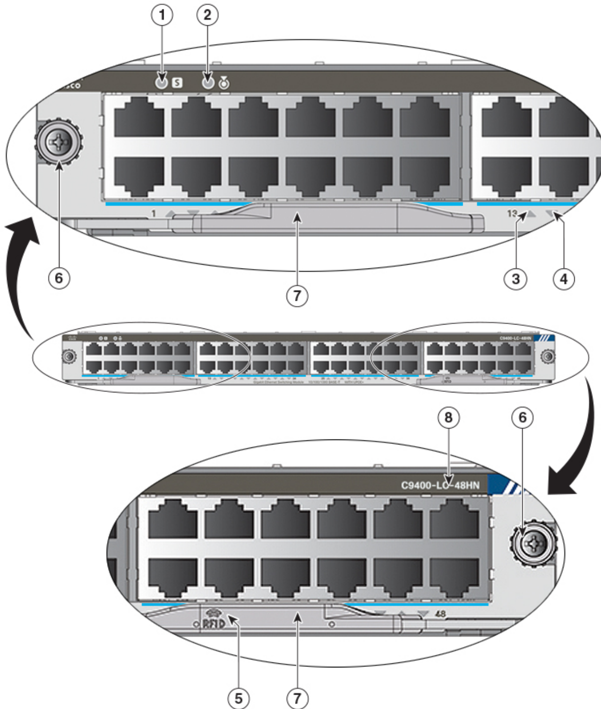
Abbildung 2: Vorderansicht der Linecard C9400-LC-48HN
