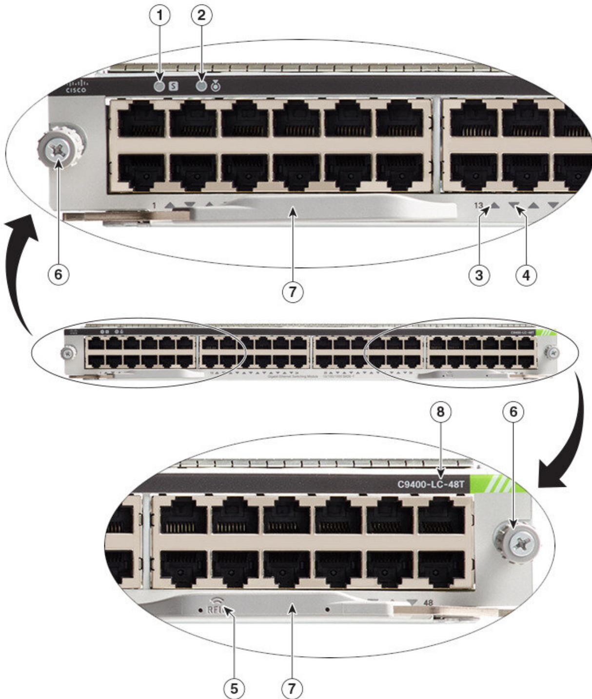
Abbildung 5: Vorderansicht der Linecard C9400-LC-48T
