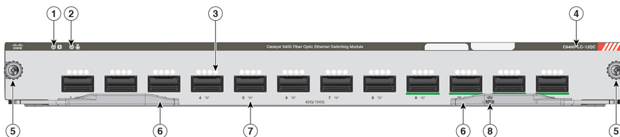
Abbildung 9: Vorderansicht der Linecard C9400-LC-12QC
