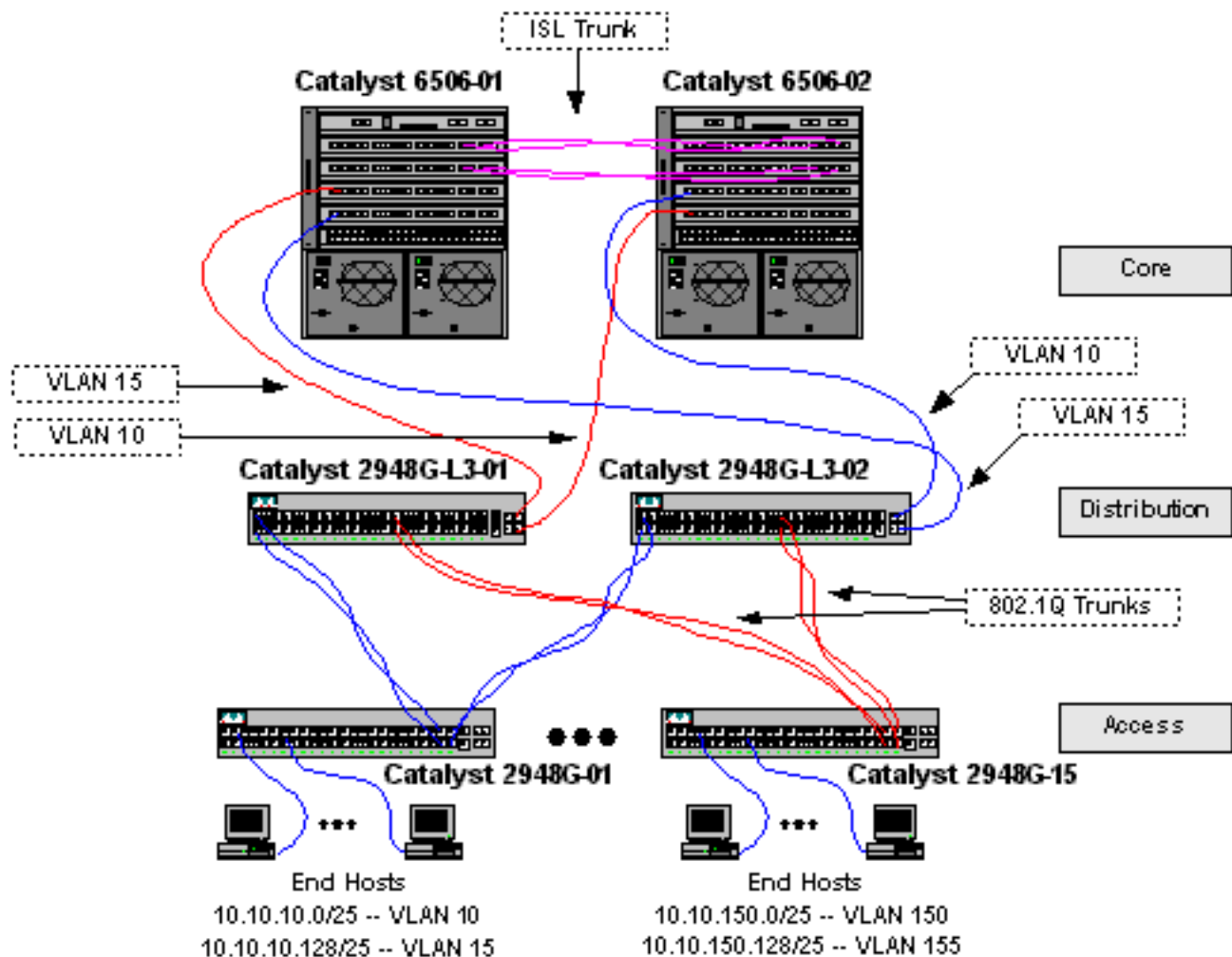
Abbildung 3: Beispiel 3 Netzwerkdiagramm
