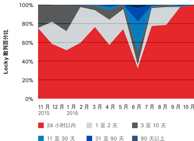
图 133 每月的 Locky 恶意软件系列的散列存活期
