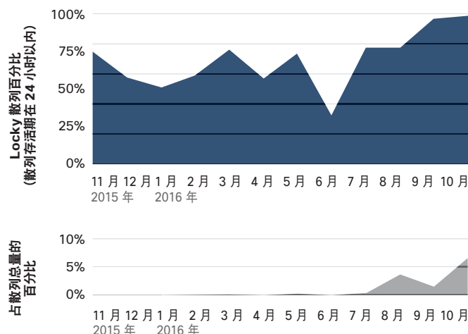
图 26 Locky 恶意软件系列的散列存活期和每月观察到的散列总量百分比
