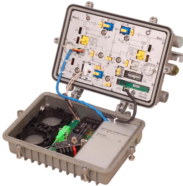
图 2. Cisco GainStar 1 GHz 光工作站壁挂
