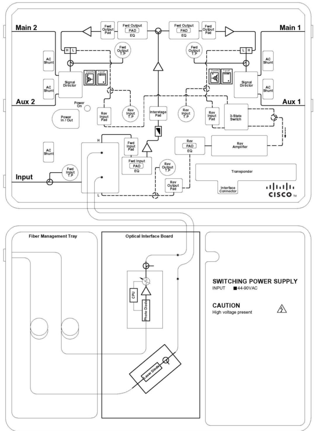
图 3. 框图
