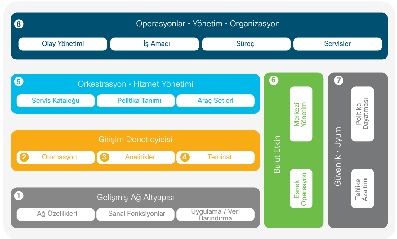
Şekil 1. Cisco DNA 8 çerçevesi
