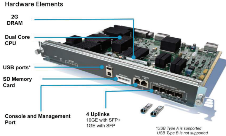
그림 1. Cisco Catalyst 4500E Supervisor Engine 7-E
