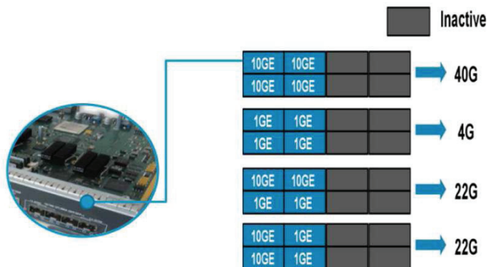
그림 2. Supervisor Engine 7-E의 고가용성 및 업링크 옵션
