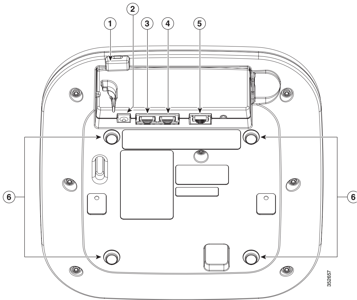
図3 アクセスポイントのポートと接続部（下部） - AIR2702E および 2702I モデル
