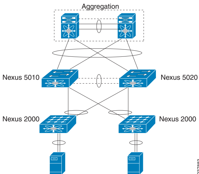
図 16 vPC ピアに直接接続されたホスト
