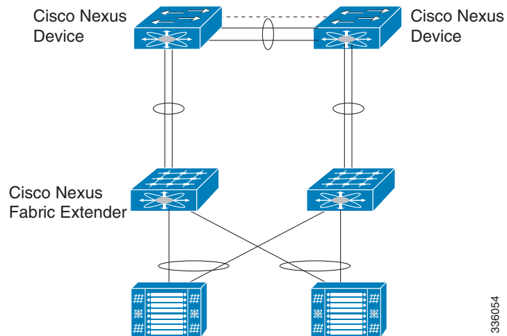
図 13 スタブ スイッチに接続されたシングルホーム FEX
