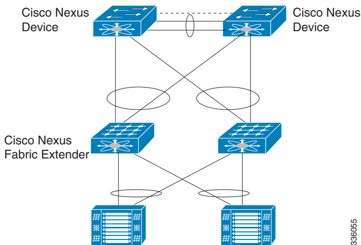
図 14 スタブ スイッチに接続されたデュアルホーム FEX
