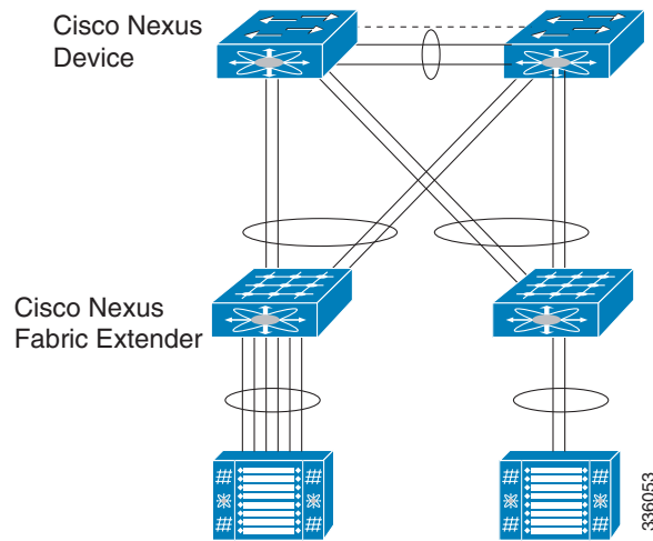
図 12 スタブ スイッチに接続されたデュアルホーム FEX
