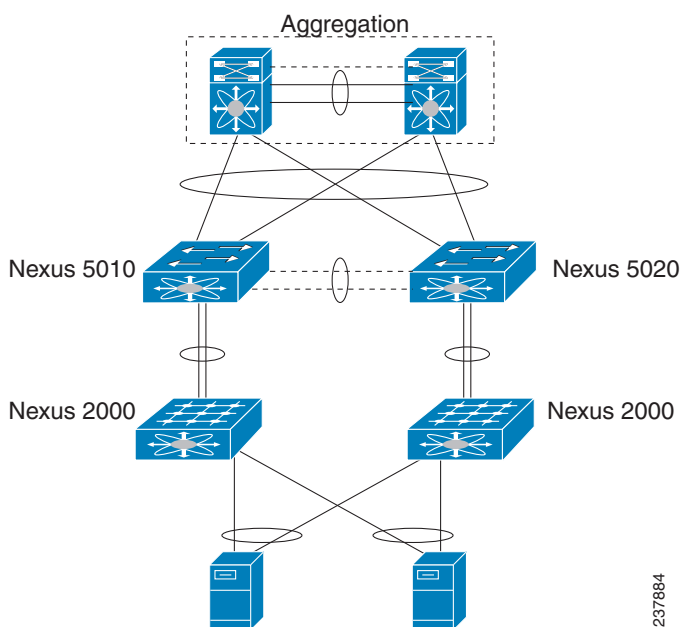
図 17 vPC がピア接続されたデュアル スーパーバイザ仮想モジュラ システムのデュアルホーム FEX とシングルホーム FEX
