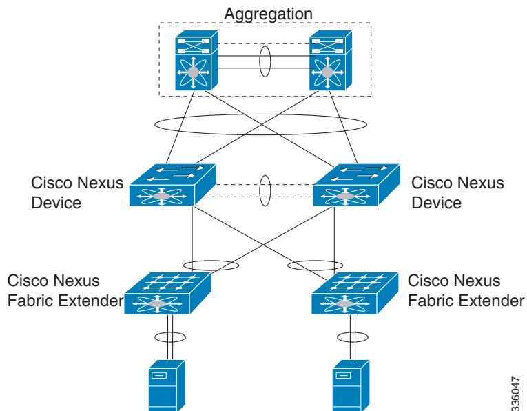
図 6 vPC がピア接続されたデュアル スーパーバイザ仮想モジュラ システムのデュアルホーム FEX
