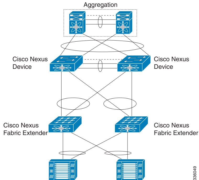
図 8 vPC がピア接続されたデュアル スーパーバイザ仮想モジュラ システムのデュアルホーム FEX
