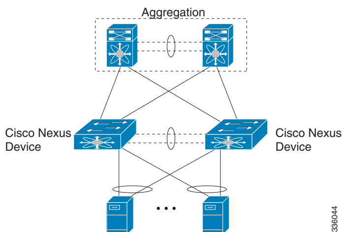
図 3 vPC ピアリング トポロジ
