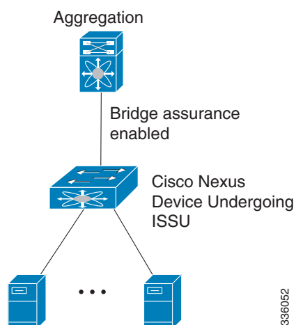
図 11 別のスイッチで Bridge Assurance を実行している Cisco Nexus デバイス
