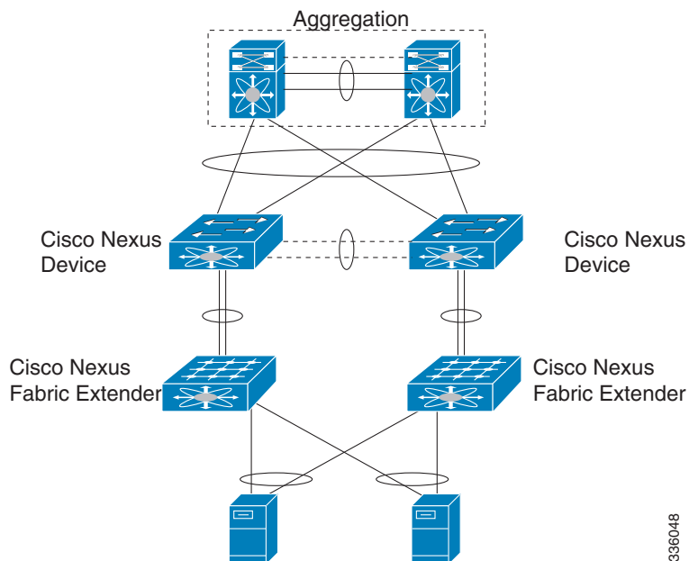
図 7 vPC がピア接続されたデュアル スーパーバイザ仮想モジュラ システムのデュアルホーム FEX とシングルホーム FEX
