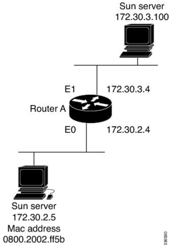
図 1: RARP サーバとしてのルータの設定
