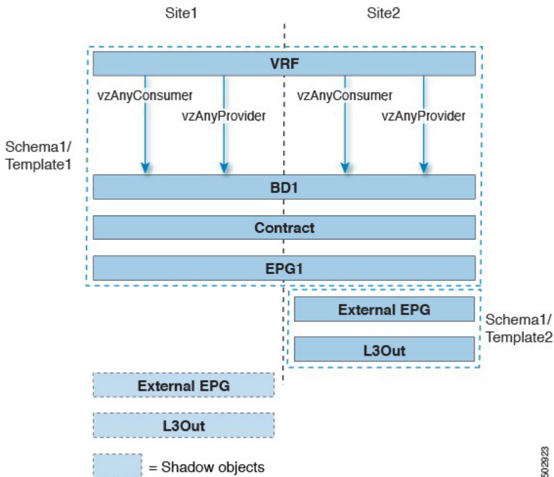
図5 VRF 内のサイト間 L3Out
