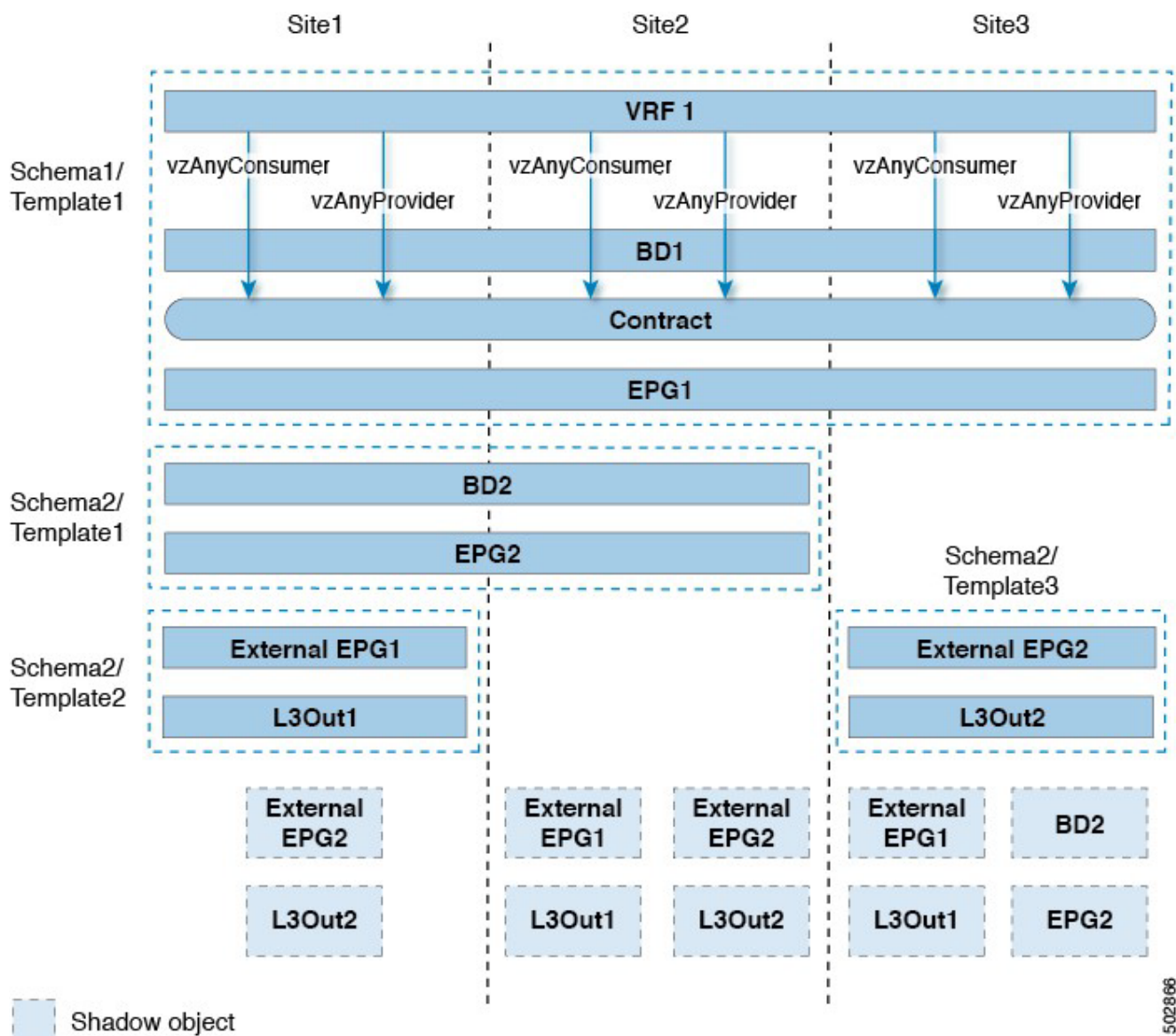
図4 サイト ローカルおよび拡張 EPG の組み合わせ
