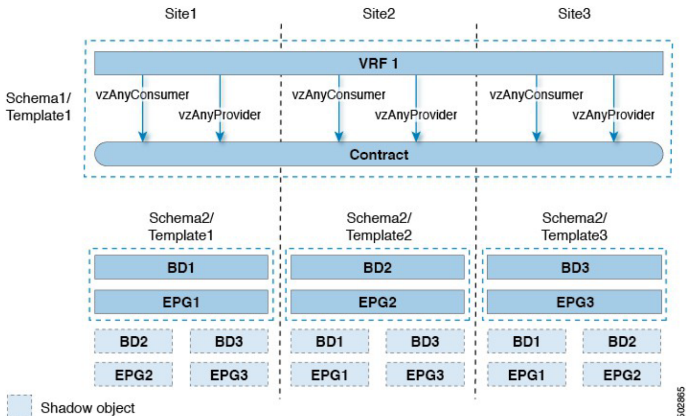
図 3. サイトローカル EPG
